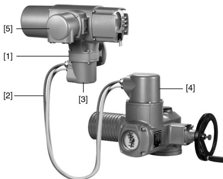
組立 図 17: 壁掛け用ブラケットへの取り付け
