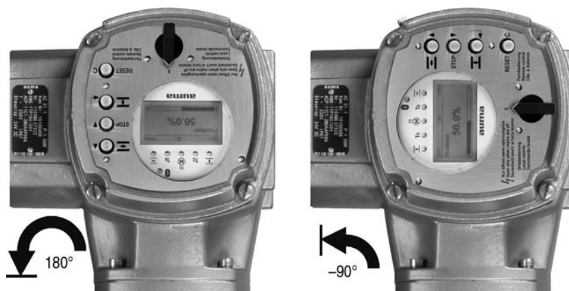
図 11: 取付位置CとD
