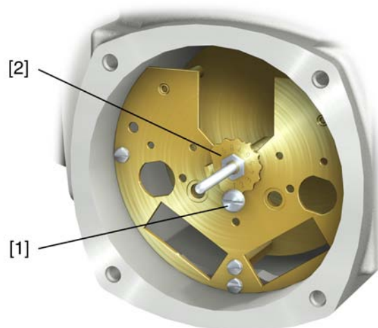
図 73: U-ギア装備のコントロールユニット
