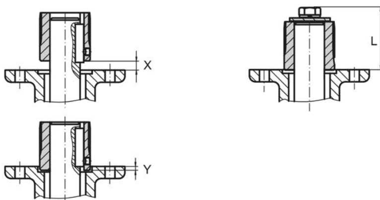
図 11: カップリングの取り付け位置
