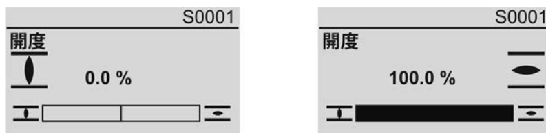
図 38: 全閉位置/全開位置に到達
