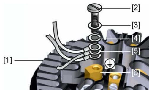
図 18: 保護アース接続部
