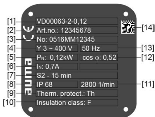
図 4: モータ銘板(例)
