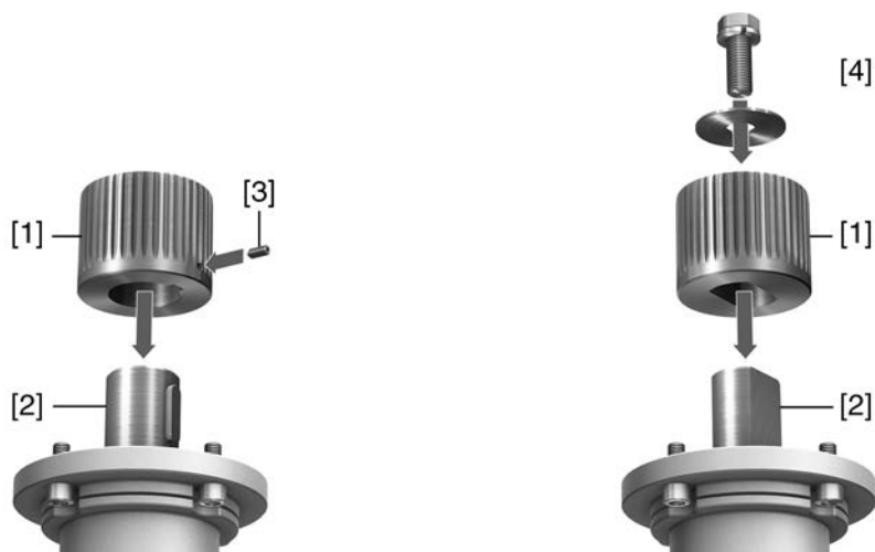
図 10: 例: カップリングの装着
