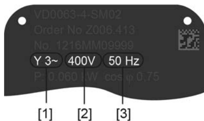
図 14: モータ銘板の例
