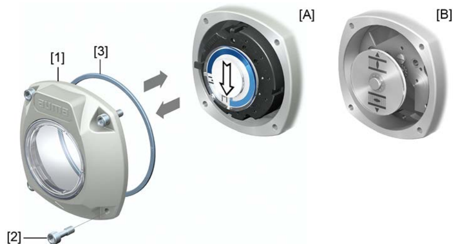
図 60: スイッチ収納部を開く/閉じる
