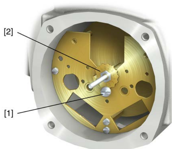
図 66: U-ギア装備のコントロールユニット
