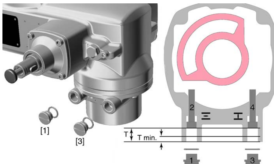
図 55: エンドストップ
