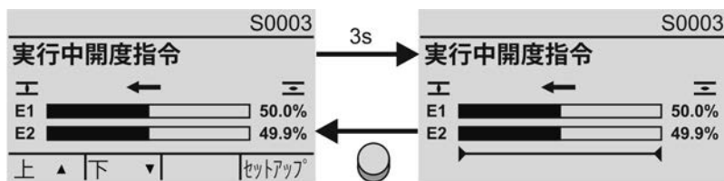
図 42: 規定値コントロール（規定制御器）の表示
