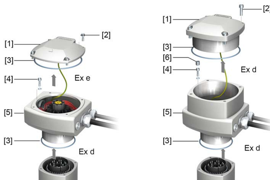
図 85: 端子板KT/KM
