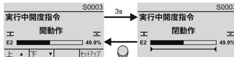
図 61: 「開 - 閉」制御の場合の表示
