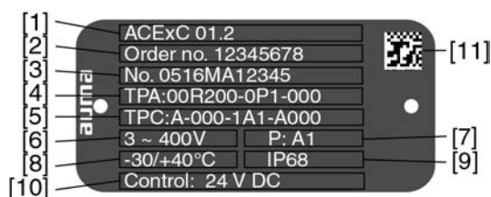
図 6: アクチュエータ制御装置銘版
