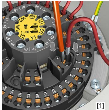
図 27: 各ケーブルを端子台に結線する
