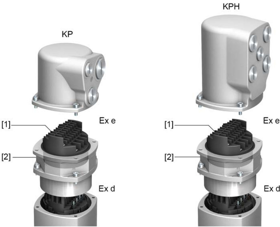
図 30: 端子板 (KP、KPH)
