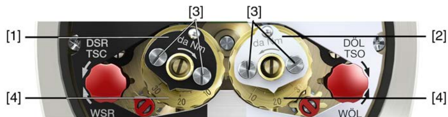
図 73: トルク測定ヘッド
