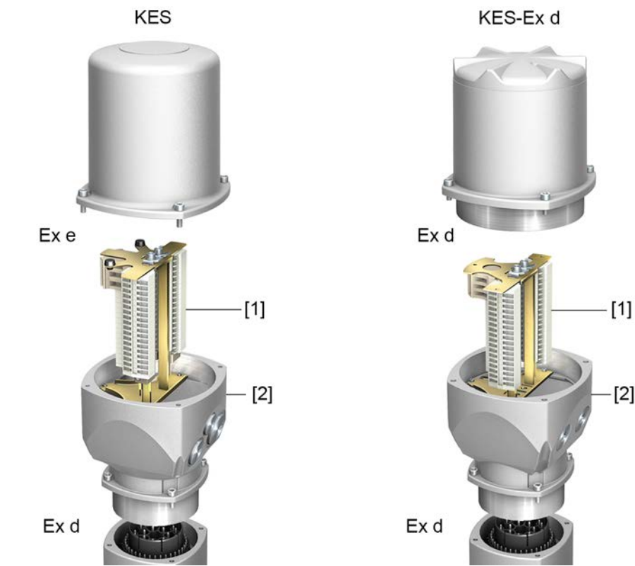
図 35: 端子板 KES
