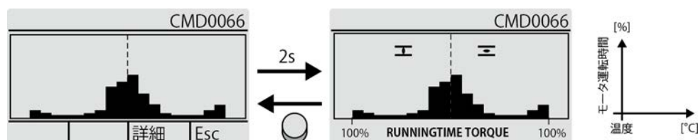
図 62: ヒストグラム「モータ運転時間-トルク」の例
