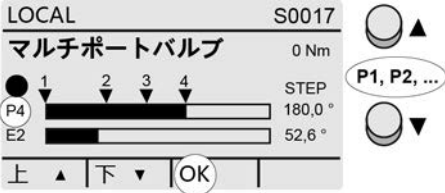
図 51: マルチポートバルブの状態表示(セクタスイッチの位置LOCAL)
