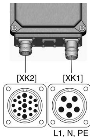
図 8: 接続の配列
