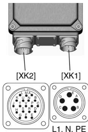
図 10: 接続の配列
