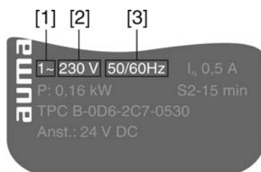
図 7: 銘板 (例)
