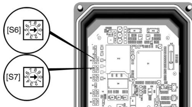
図 24: シーティングトルクのスイッチ
