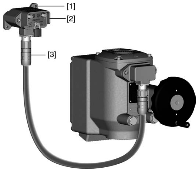
図 17: 壁掛け用ブラケットの現場操作機 での構成
