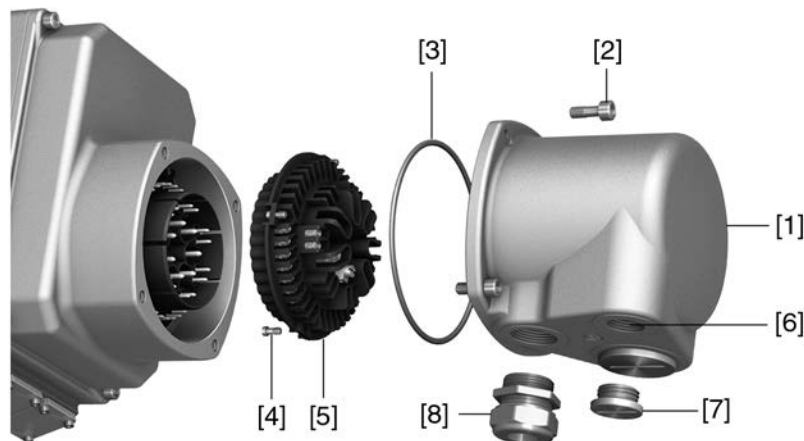
図 13: AUMAプラグソケットコネクタ 接続、型式 S
