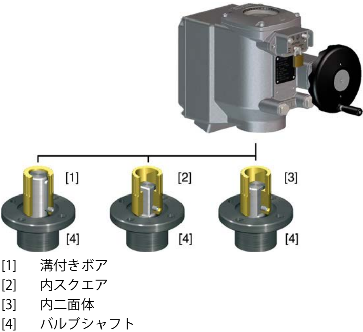
図 5: カプリングバージョン
