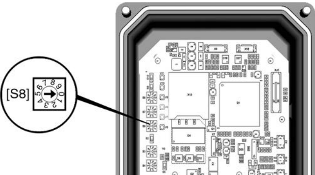
図 25: 回転数のスイッチ
