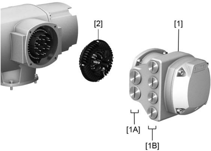
図 18: 端子板SD
