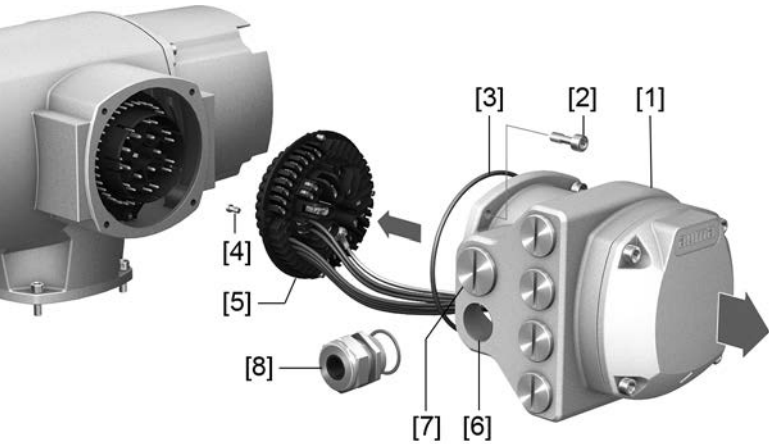
図 19: 電源接続空間を開く
