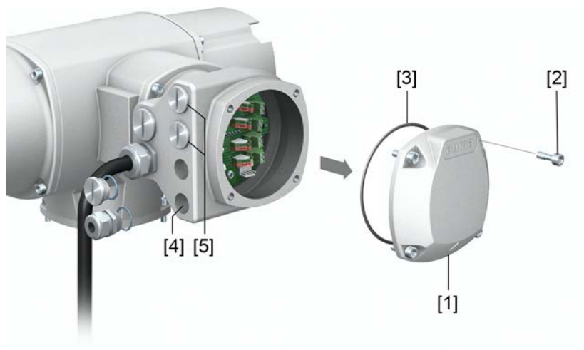
図 23: フィールドバス端子箱カバーを開く
