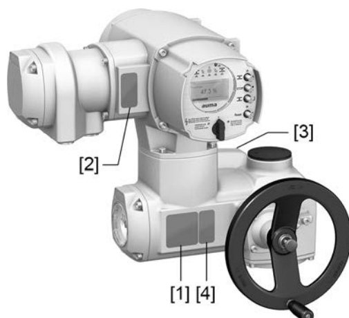
図 1: 銘板の取り付け位置
