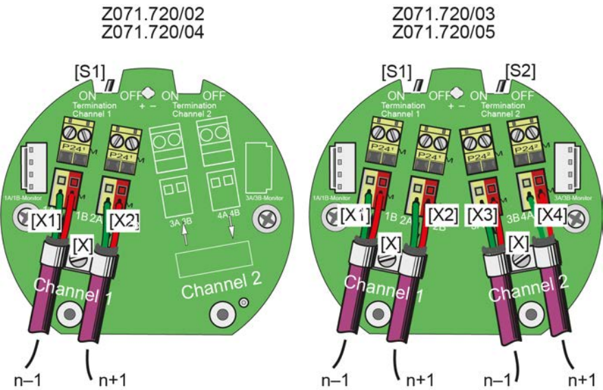
図 25: 接続ボードのバリエーション
