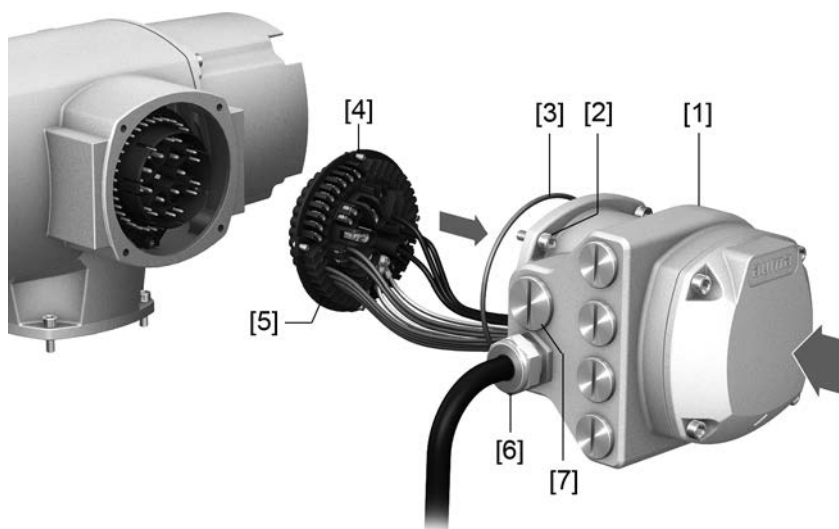
図 22: 電源接続空間を閉める
