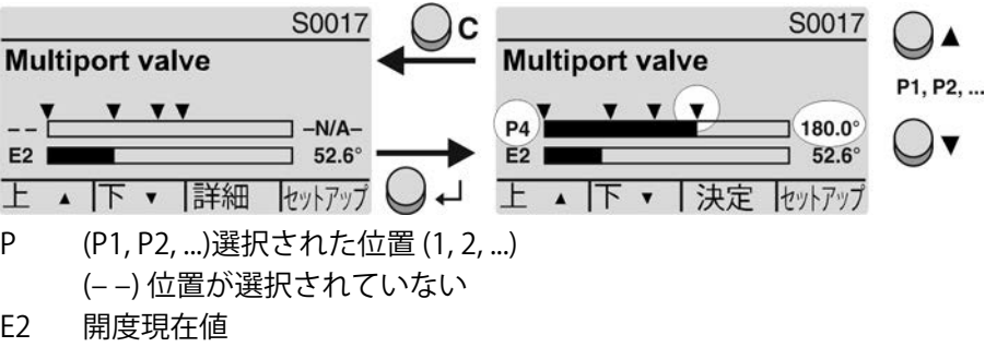
図 53: マルチポートバルブのステータス表示 (例 P4 = 180° C)
