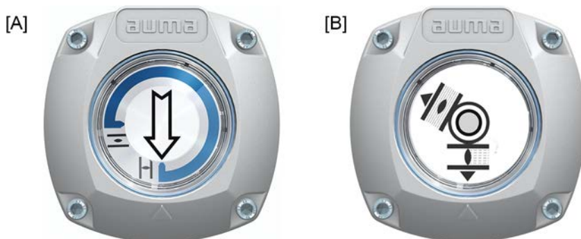
[A] 機械式開度表示（自己調整型）
