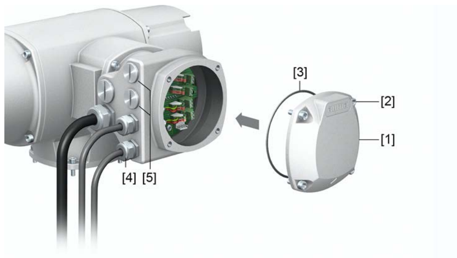
図 26: フィールドバス端子箱を閉じる
